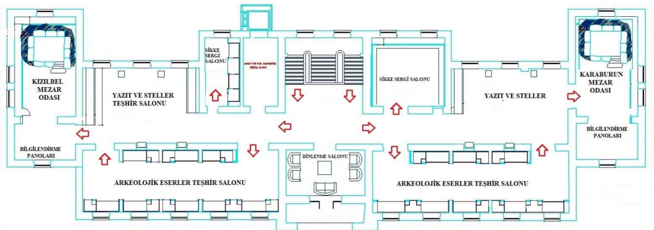
Antalya Elmalı Müzesi Müdürlüğü 1. Kat Planı
