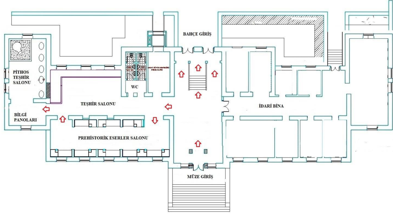
Antalya Elmalı Müzesi Müdürlüğü Zemin Kat Planı
